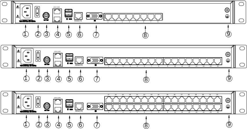
后视图
