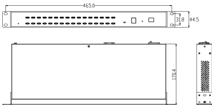
图 1-1.2 尺寸图
